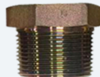
42.46 มม 11.5G
